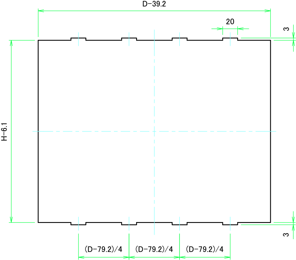
Dパネル1表面 / D Panel 1 Frontside
