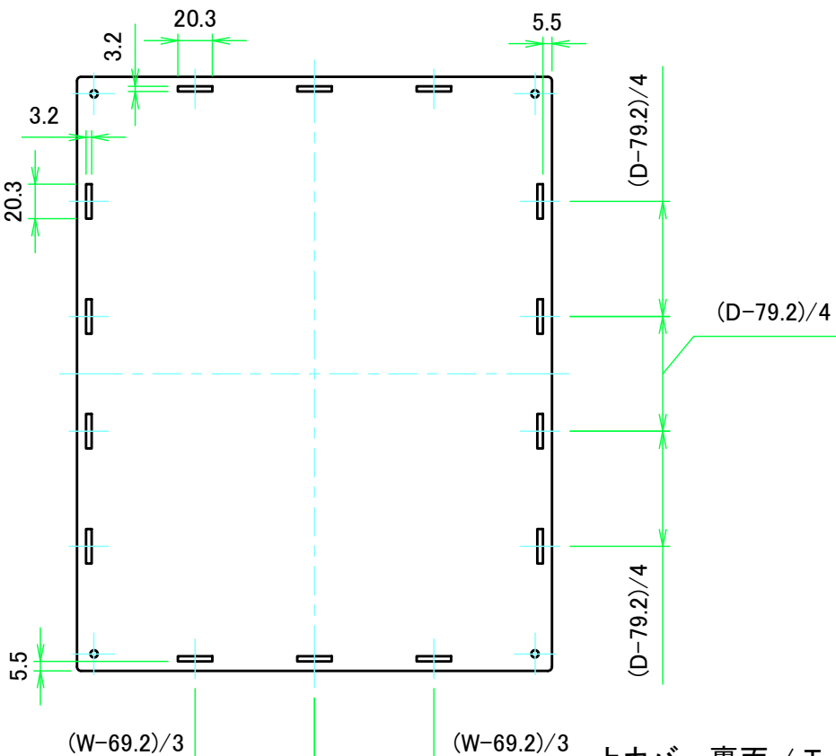
上カバー裏面 / Top cover Backside
